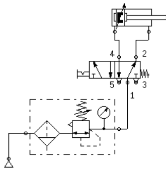
Gambar Rangkaian Pneumatic
